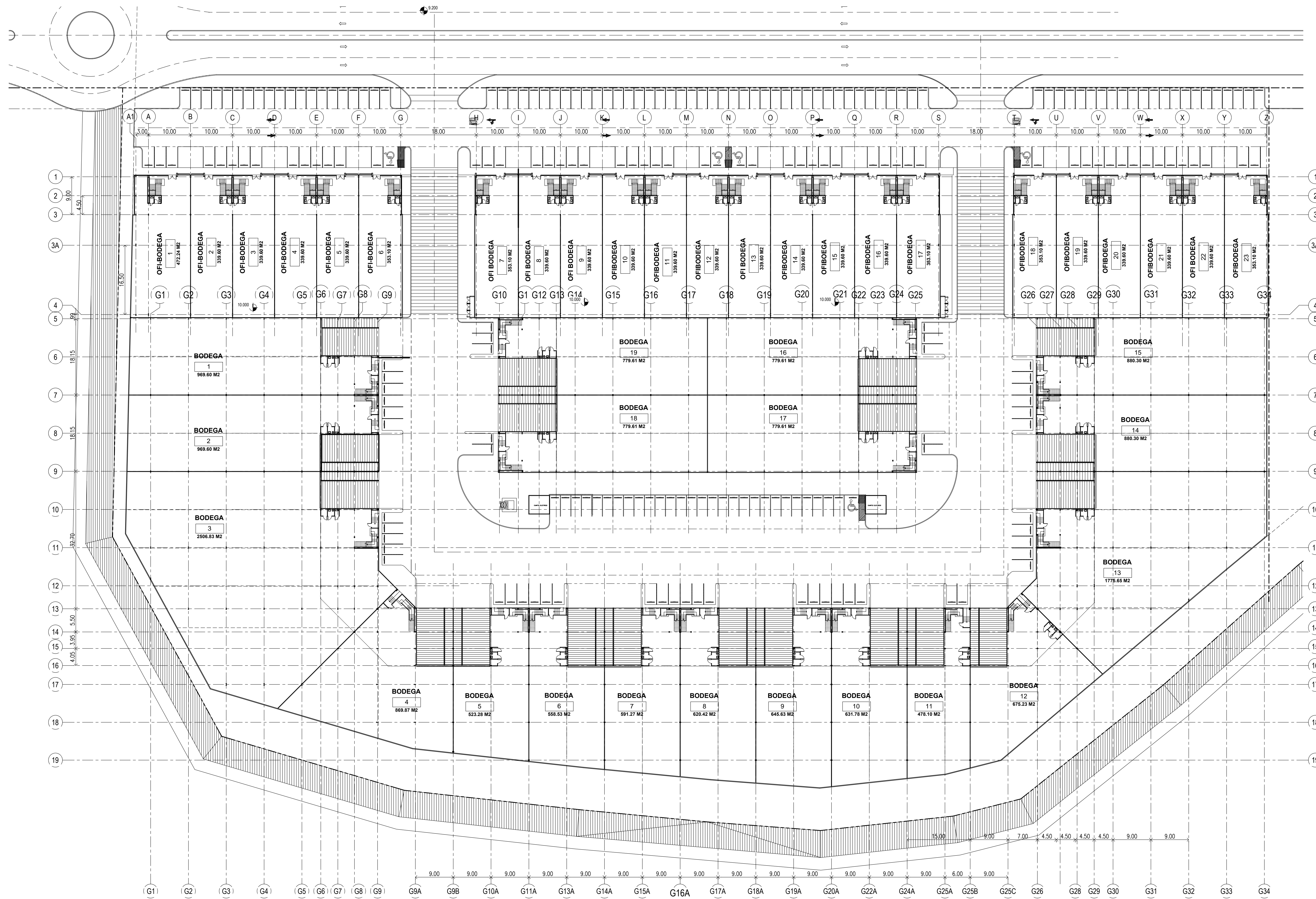
PLANTA ARQUITECTONICA BAJA GENERAL ESCALA 1:400
