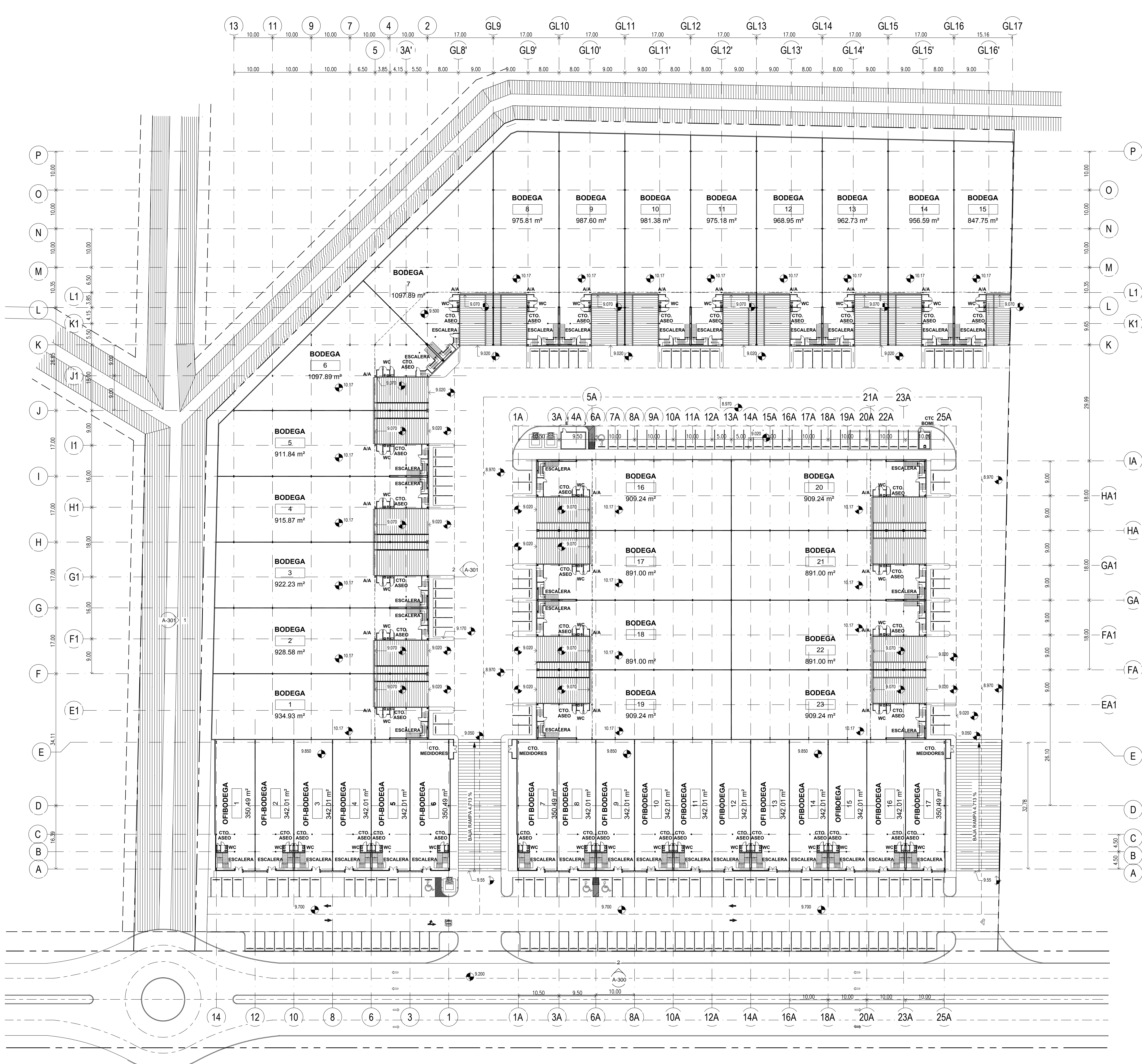
PLANTA ARQUITECTONICA BAJA - GENERAL ESCALA 1:400
