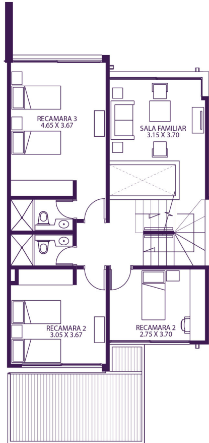
Nivel 02
