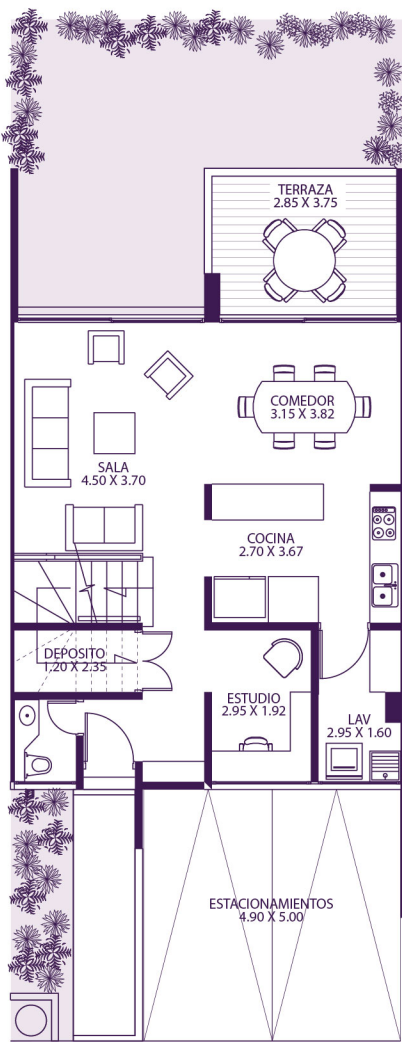
Nivel 01
