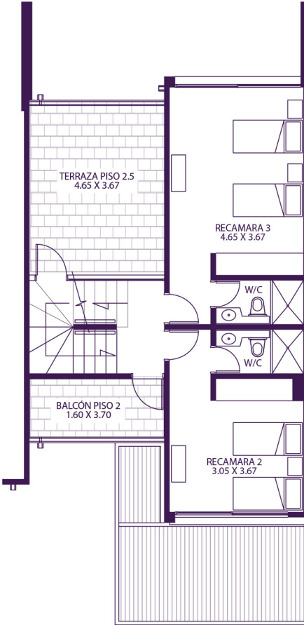
Nivel 02
