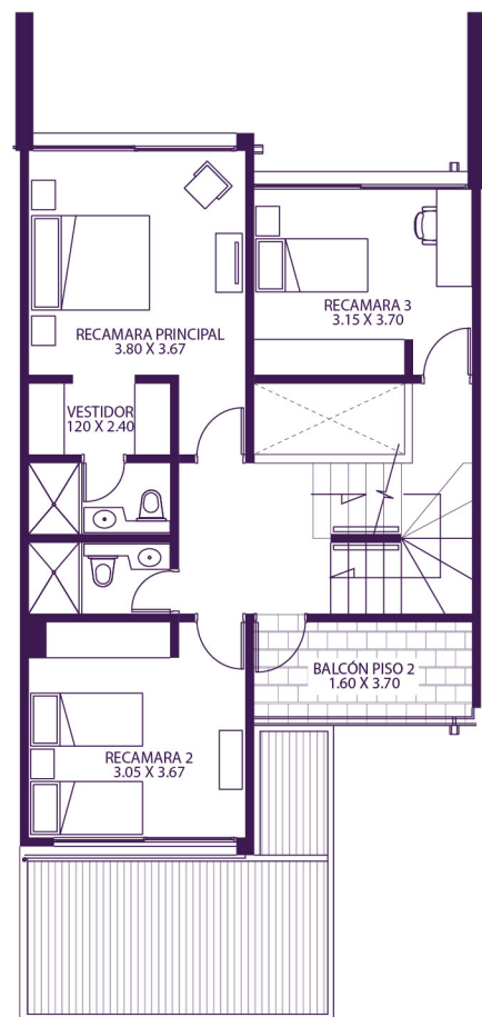
Nivel 02
