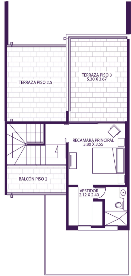
Nivel 03
