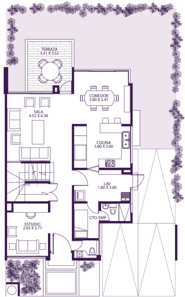
Nivel 01
